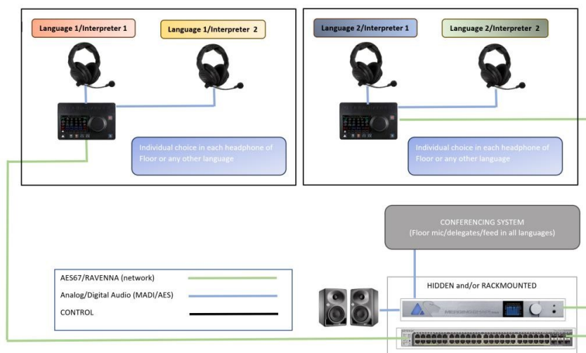
Merging Technologies 口译解决方案示意图
